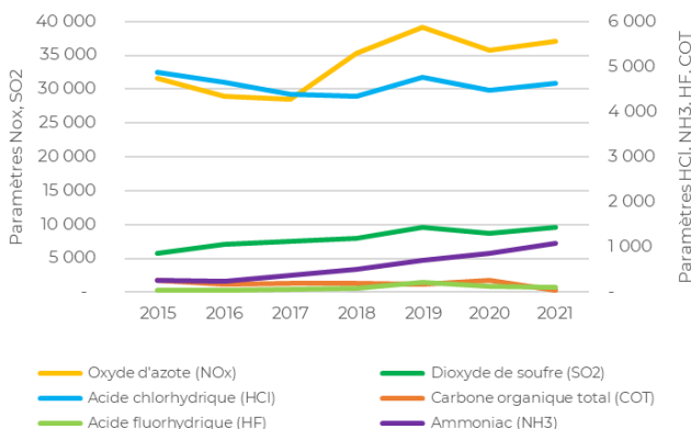
Contrôle des rejets atmosphériques (mesures en flux - cumul sur les 2 lignes) en kg
